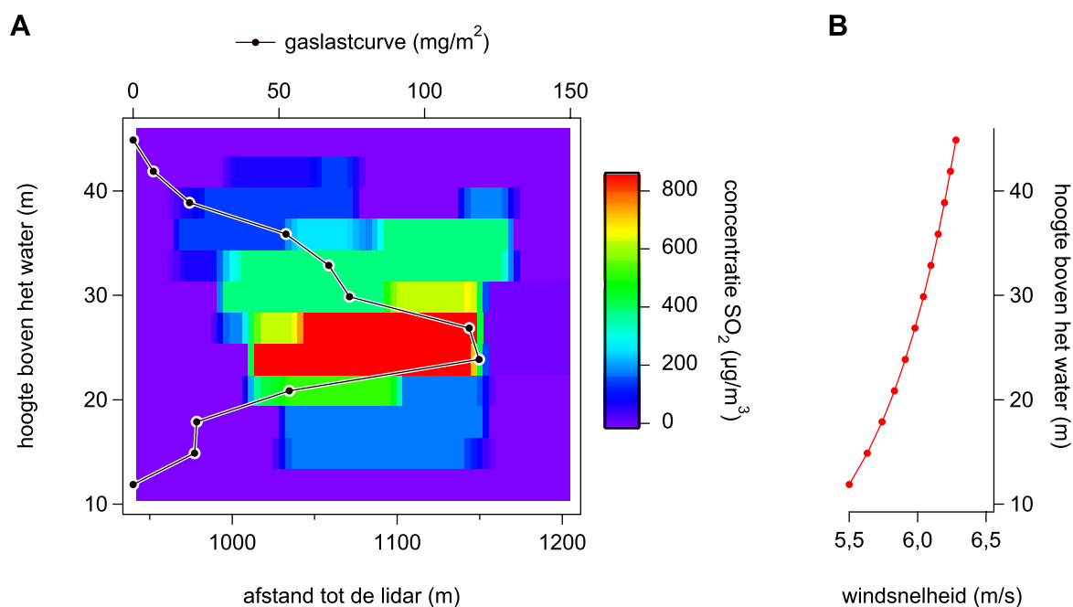
Figuur 2-7. A: uitsnede uit Figuur 2-6 van de rookpluim van de HMS Rotterdam, en de bijbehorende gaslastcurve. B: logaritmisches windprofiel.
