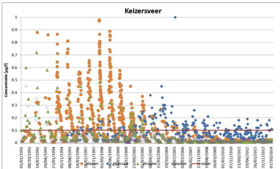
Figuur 1 Concentraties van simazine (grijs), diuron (oranje), atrazine (groen) en glyphosaat (blauw) op het drinkwaterinnamepunt Keizersveer van 1991 tot 2014. De rode lijn geeft de oppervlaktewaternorm op drinkwaterinnamepunten weer (0,1 µg/L).
