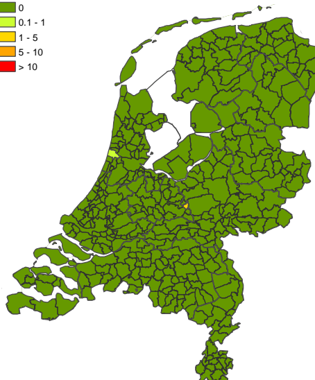
Figuur 2 Overschrijdingen PM 10 van de etmaalnrm in 2016 getoetst aan de grenswaarde (links). In de rechterfiguur worden de resultaten gepresenteerd met bandbreedte. Exclusief overschrijdingen bij veehouderijen.
