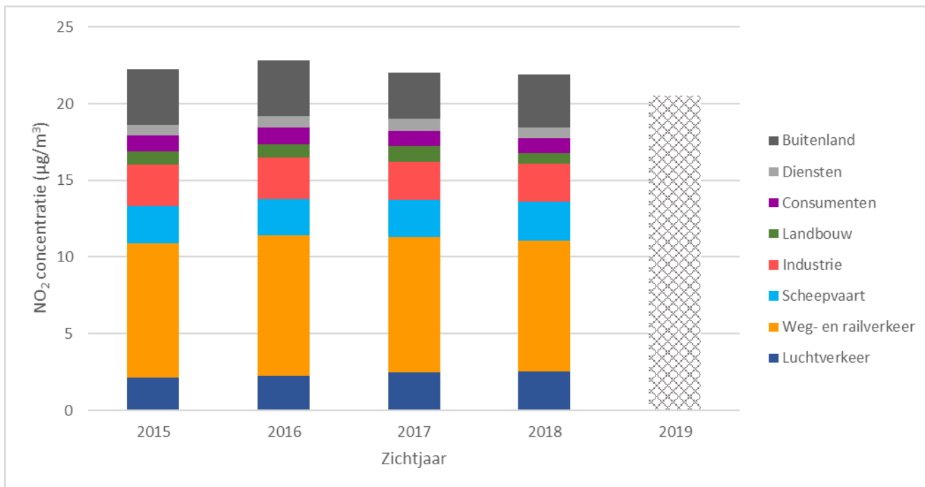
Figuur 3 Bijdrage per sector aan de jaargemiddelde NO 2 -concentratie in het studiegebied voor de verschillende zichtjaren (voor 2019 is alleen de totale concentratie getoond).
