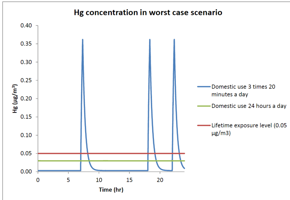
Figuur 1 Gemodelleerde concentratie kwik (Hg) in de ruimte ( 15 \text{ m}^3 ) gedurende een dag voor een worst-case gasconsumptiepatroon met een ventilatievoud van 2,5 vervangingen/uur (gekopieerd uit NAM, 2014)
