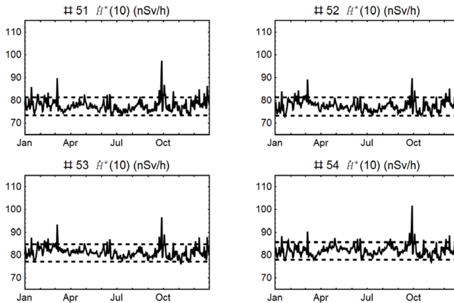
Figuur 4 Het daggemiddelde omgevingsdosisequivalenttempo \dot{H}^*(10) voor de MONET-monitoren M51-M54 aan de terreingrens van COVRA in 2020 samen met, als gestippelde lijnen, de variatie van de natuurlijke achtergrond.
