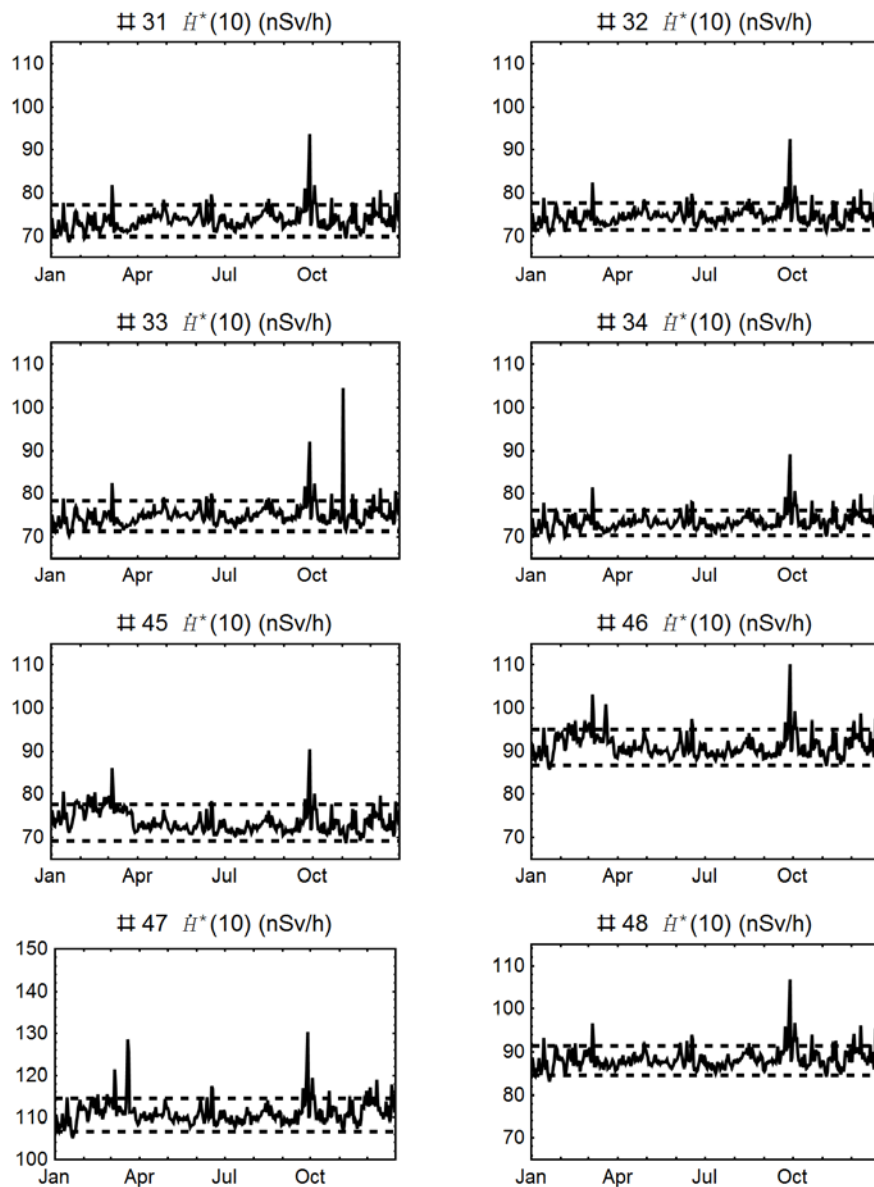
Figuur 3 Het daggemiddelde omgevingsdosis-equivalenttempo \dot{H}^*(10) voor de MONET-monitoren M31-M34 en M45-M48 aan de terreingrens van COVRA in 2020 samen met, als gestippelde lijnen, de variatie van de natuurlijke achtergrond. De figuur voor monitor 47 heeft een andere schaalverdeling voor de y as.
