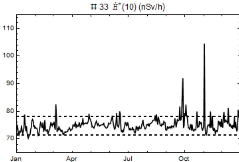
Figuur 5 Het gemeten omgevingsdosisequivalenttempo voor monitor 33 in 2020 (uit Figuur 3) samen met de natuurlijke achtergrond en de spreiding als gestippelde lijnen over het jaar. De pieken op 17 juni, op drie dagen in september (23, 27 en 28 september) vallen samen met hevige neerslag. De verhoging op 2 november is mogelijk veroorzaakt door het transport van nucleair materiaal (afvoer splijstofelementen).
