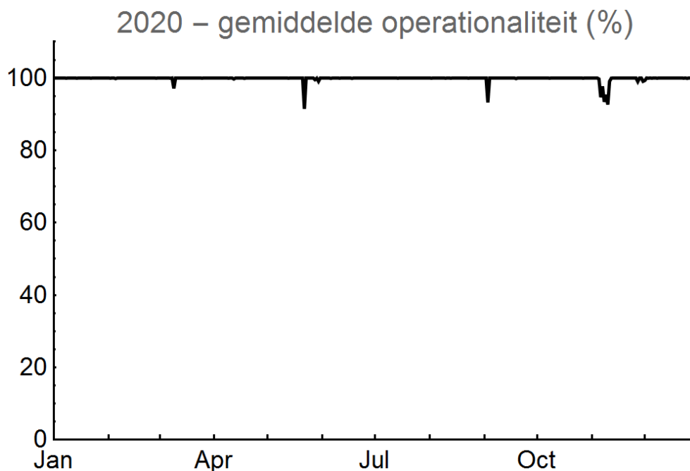
Figuur 2 Gemiddelde operationaliteit per dag van MONET aan de terreingrens van COVRA in 2020.
