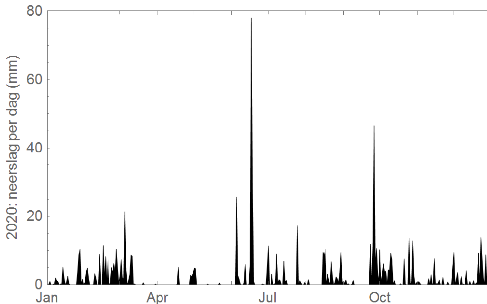
Figuur 6 Neerslag per dag, in mm, gemeten door het KNMI weerstation van Vlissingen (bron: KNMI). Hevige neerslag op 17 juni, 23 en 28 september 2020 valt samen met een verhoging van het omgevingsdosisequivalenttempo van alle monitoren van het MONET-meetnet.
