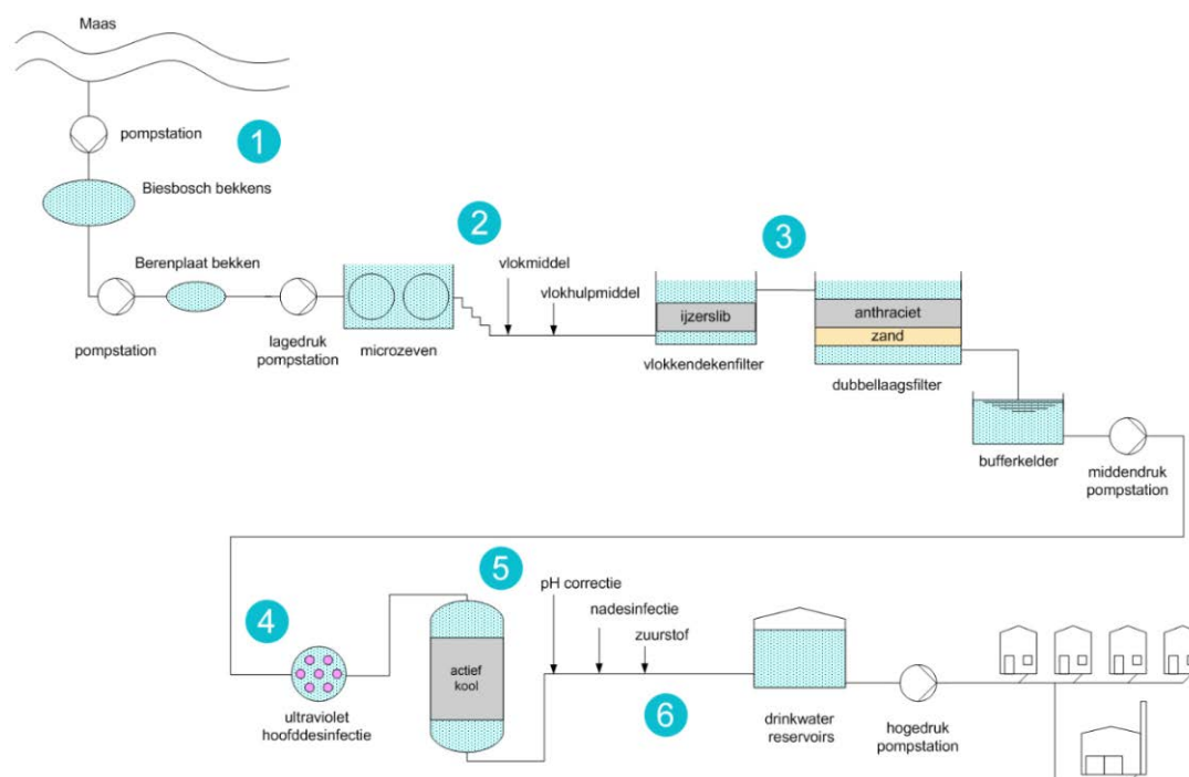
Figuur B5.2. Zuiveringsproces van productiebedrijf Berenplaat van Evides (Evides, 2016)
