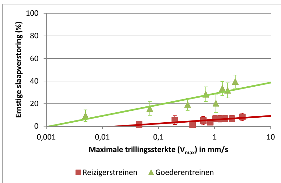
Figuur 4.12 Relatie tussen blootstelling aan trillingen door respectievelijk reizigers- en goederentreinen in V_{max} en zelfgerapporteerde ernstige slaapverstoring door trillingen van deze treinen. Ook is per spoorbron de prevalentie van (met 95% betrouwbaarheidsinterval) van ernstige slaapverstoring per deciel te zien.
