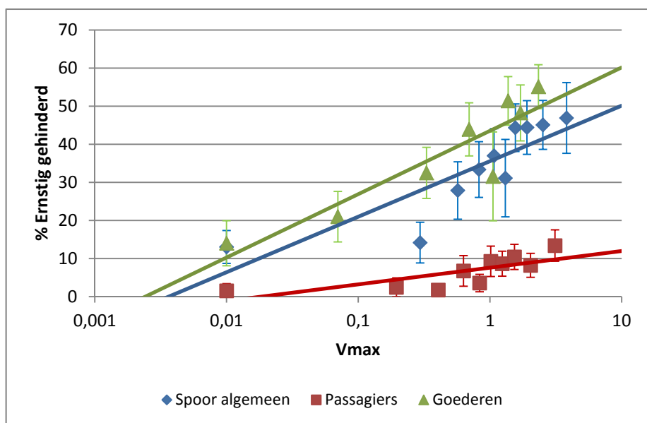
Figuur 4.8 De relatie tussen de blootstelling aan trillingen van respectievelijk treinverkeer, reizigerstreinen en goederentreinen ( V_{max} ) en het aandeel van de populatie dat ernstige hinder door trillingen van deze treinen ervaart. Ook is per spoorbron de prevalentie (met 95% betrouwbaarheidsinterval) van ernstige hinder per deciel te zien.
