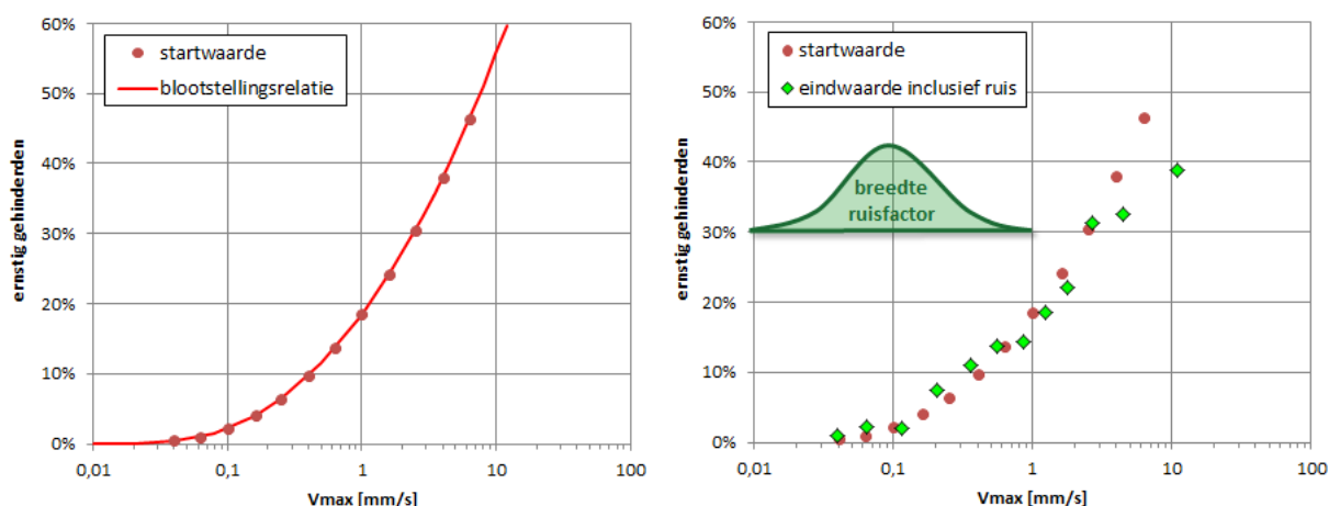
Figuur B8.2 Simulatie van het effect van het toevoegen van een ruisfactor van 0,1 tot 10 in V_{max} .
